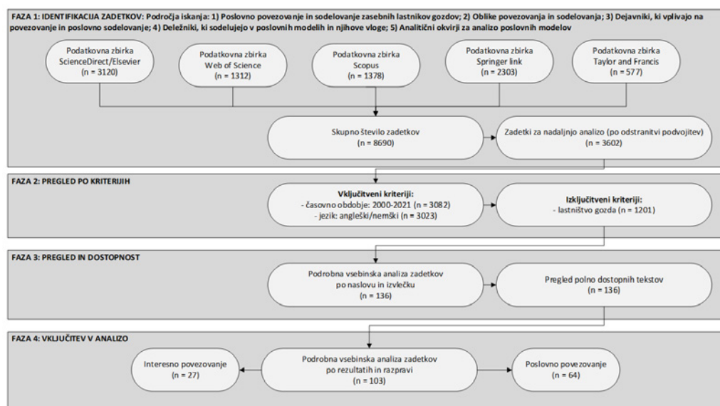
Slika 1: Shematski prikaz poteka pregleda literature po metodologiji PRISMA.
