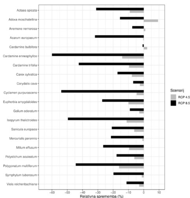
Slika 1: Relativna sprememba (%) skupne površine z verjetnostjo pojavljanja nad 0,5 za posamezno rastlinsko vrsto in podnebni scenarij (RCP 4.5 – sivi stolpci, RCP 8.5 – črni stolpci) za območje Evrope.
